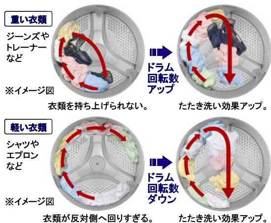
[図 2 「センサービッグドラム洗浄」]
