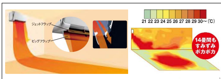
〔図 8 「ビッグフラップ」と「ジェットフラップ」で床面を暖房〕
