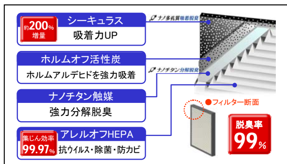
[図3 ナノテク BIG HEPA フィルターの構成]
